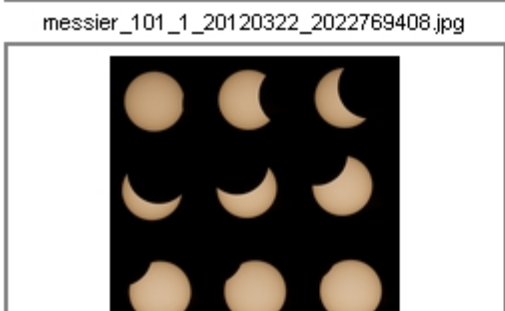
anfinsternis_20_maerz_2015_20150326_15470209C
