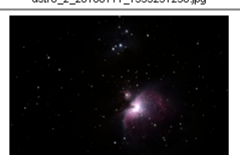
grosser_orionnebel_1_20120313_1162531484.jpg
