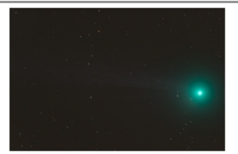
2014_q2_20150116_1306163123.jpg
